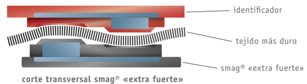
corte transversal smag® «extra fuerte»
