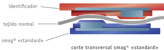
corte transversal smag® «standard»
